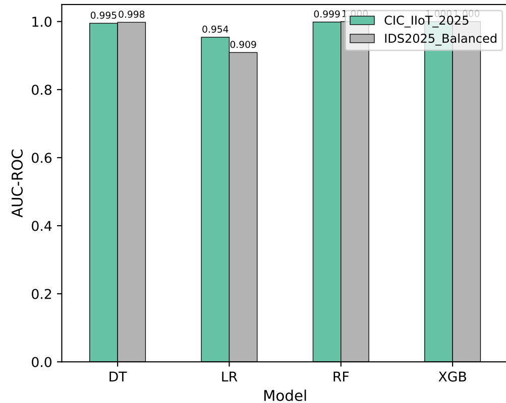
AUC-ROC
