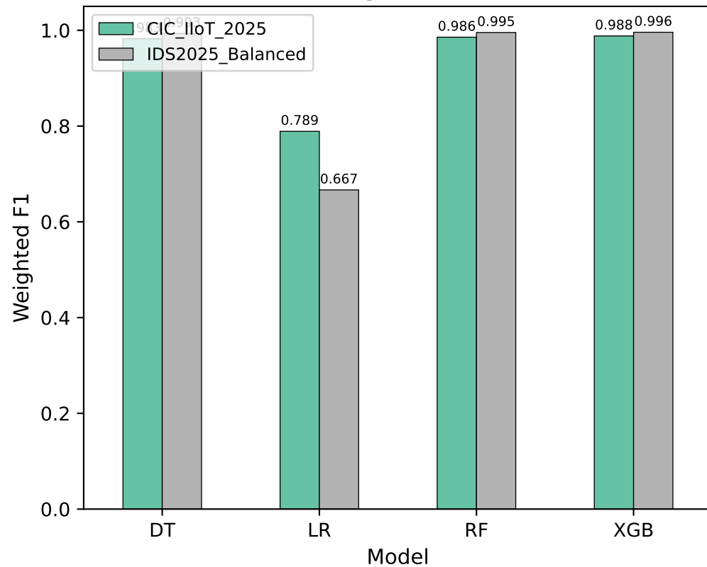
Weighted F1
